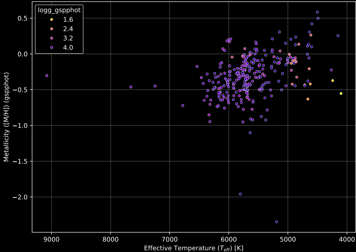
GALAH DR4 Field: [434] Stellar Population Parameters (n= 270)
