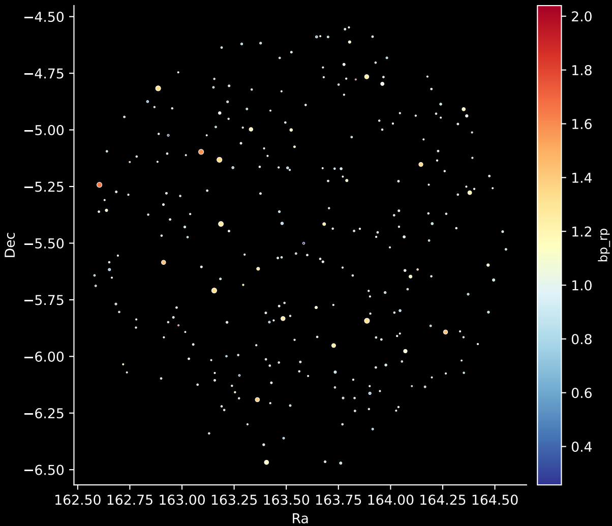
GALAH DR4 Field: [434] Stars: 270
